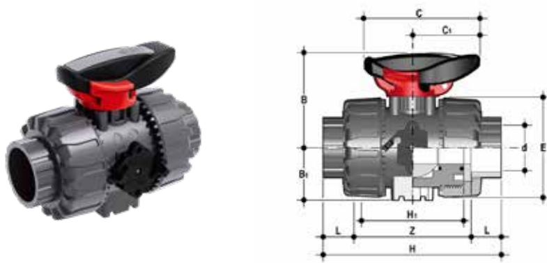
Valvola a sfera a due vie DUAL BLOCK® con attacchi femmina per incollaggio, serie metrica
