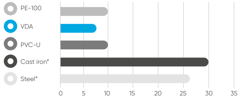
Weight per meter kg/m
